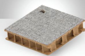
Tela de arpillera adherida a estructura panal de cartón
