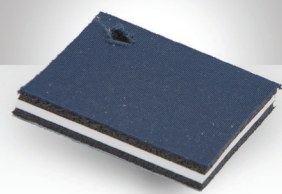
Tela adherida a caucho adherido a lámina de PVC
